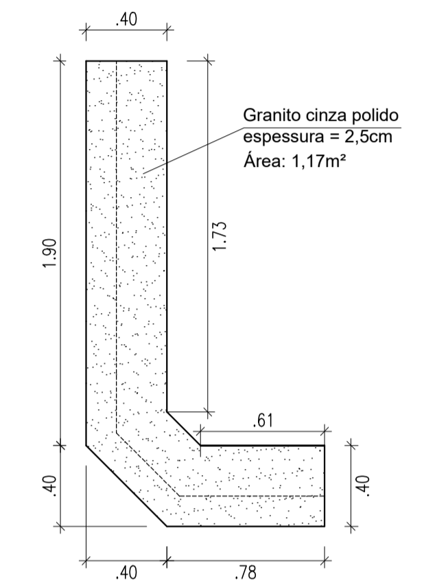
DETALHE BALCÃO - VISTA SUPERIOR ESC.:1:25
