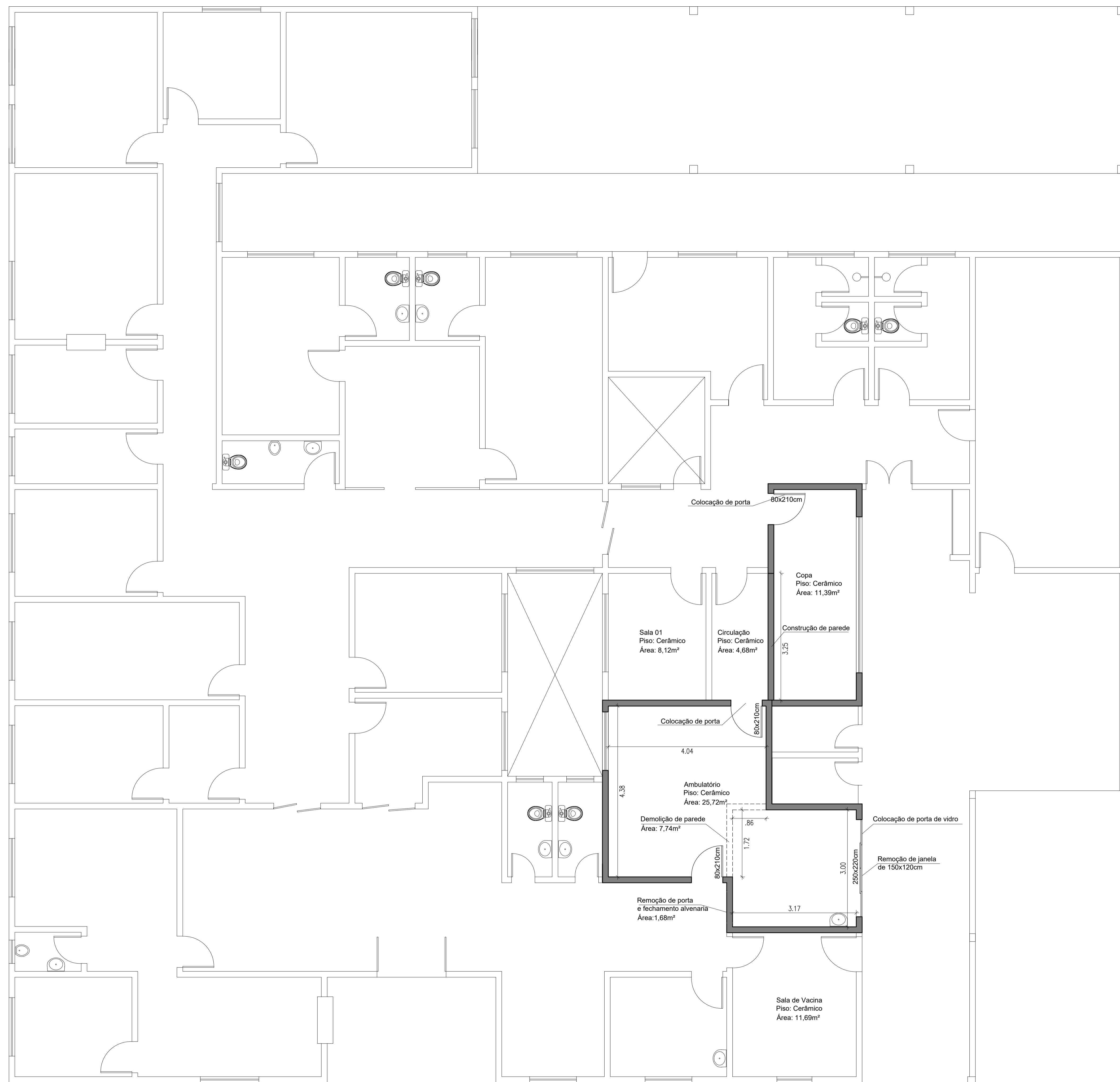
PROJETO REFORMA AMBULATÓRIO ESC.:1:50
