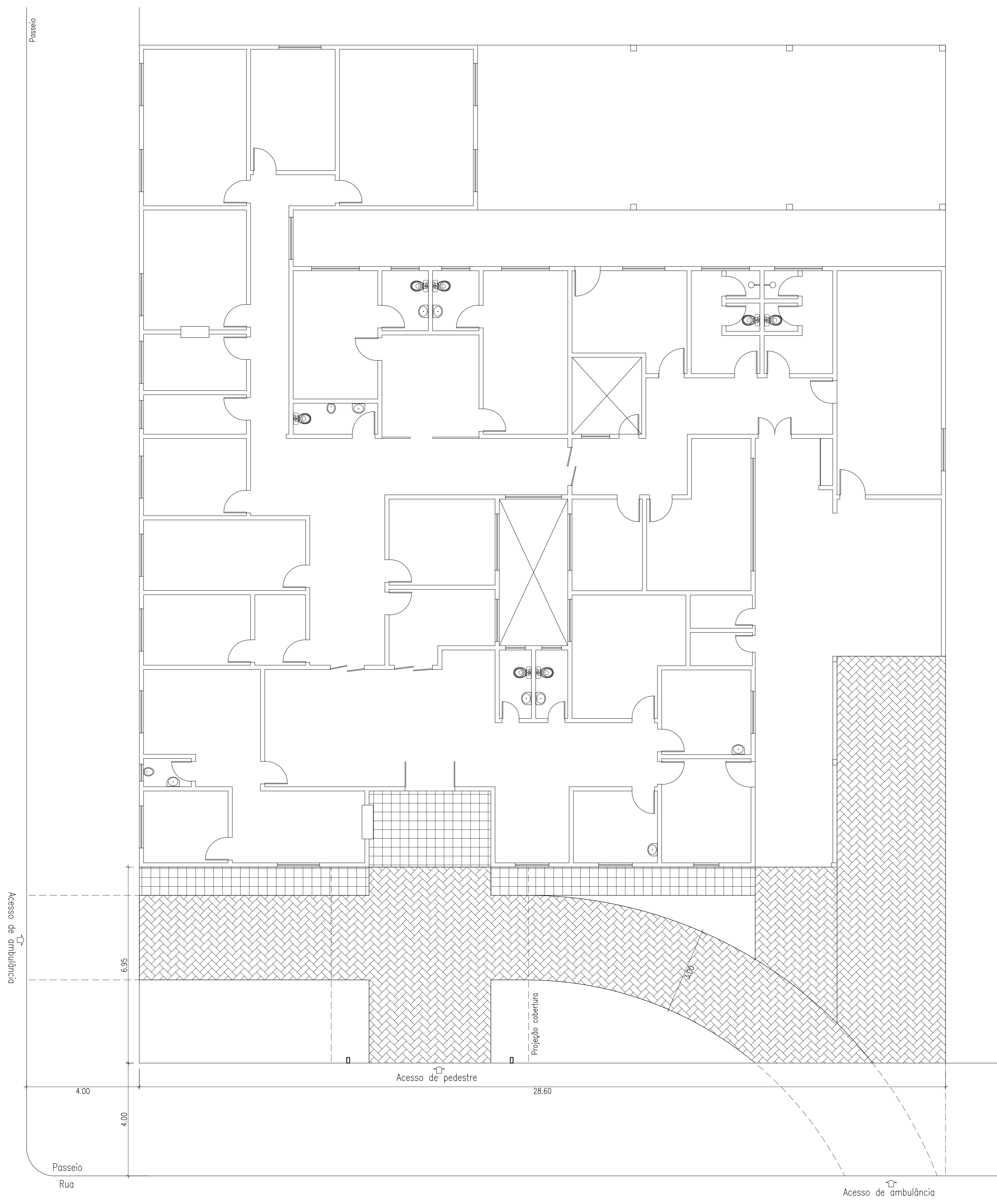
PROJETO LOCAÇÃO PAVIMENTAÇÕES EXTERNAS ESC.:1:100
